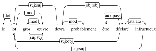
FIGURE 1 – Exemple d’analyse en dépendances surfaciques (arcs au-dessus de la phrase) et en dépendances profondes (combinaison des arcs pleins du dessus et des arcs en dessous) repris de Candito et al. (2014) . Le mot "être" n’est pas présent dans l’analyse en dépendances profondes et il existe un cycle contenant "gros" et "œuvre".
